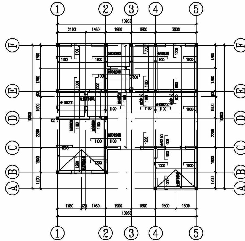
坡屋面板配筋图
