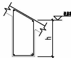
水平梁交坡屋面大样
