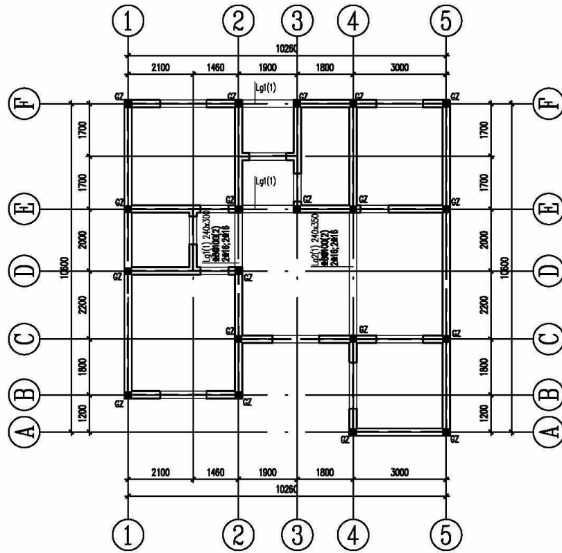
坡屋面结构布置图
